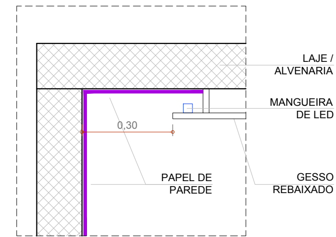
DETALHE 03 SANCA ILUMINADA ESCALA 1:25
