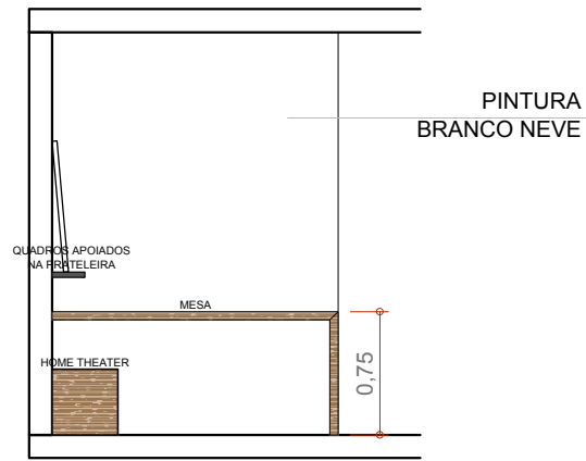
VISTA 02 ESCALA 1:50
