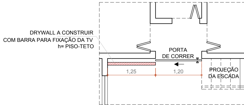
PLANTA ESCALA 1:50
