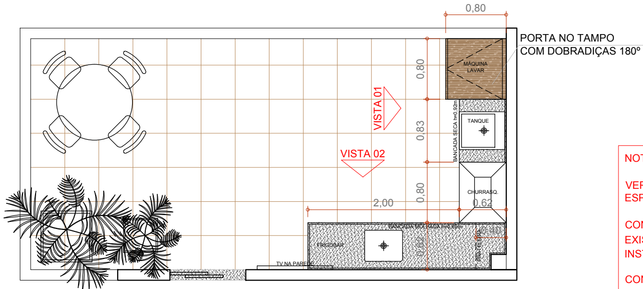
PLANTA ÁREA EXTERNA ESCALA 1:50
