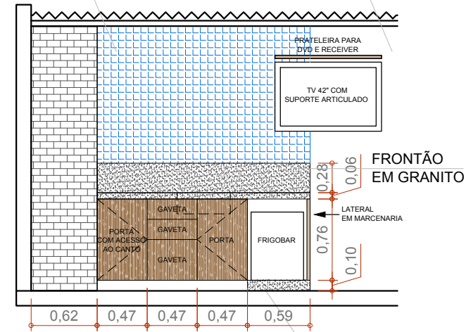
VISTA 02 ESCALA 1:50
