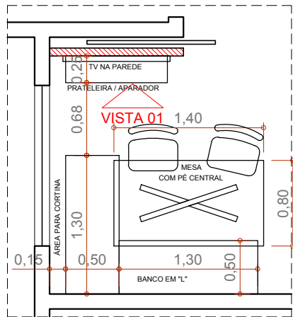
PLANTA ESCALA 1:50
