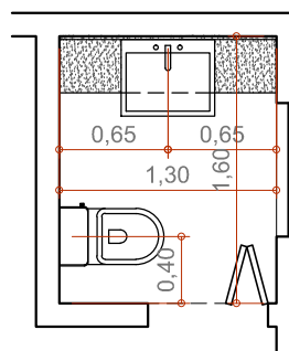
PLANTA LAVABO ESCALA 1:50
