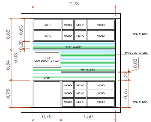
VISTA 03 ESCALA 1:50
