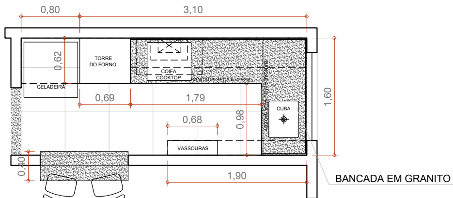
PLANTA COZINHA ESCALA 1:50
