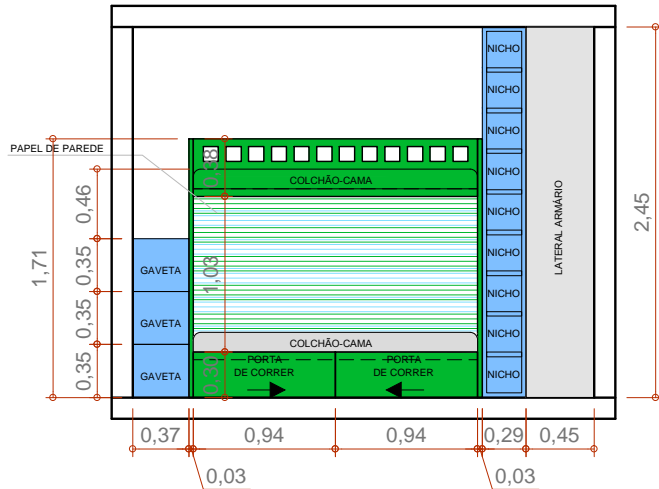
VISTA 01 ESCALA 1:50
