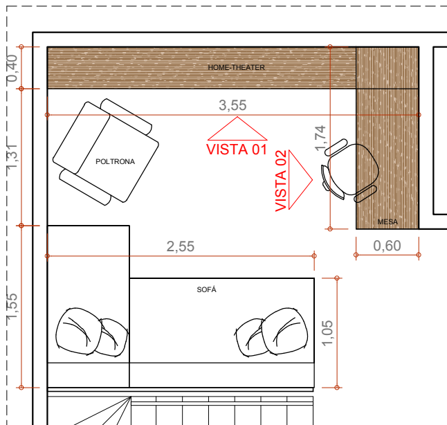
PLANTA ESCALA 1:50
