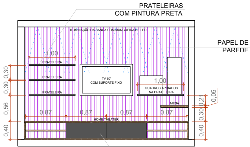
VISTA 01 ESCALA 1:50
