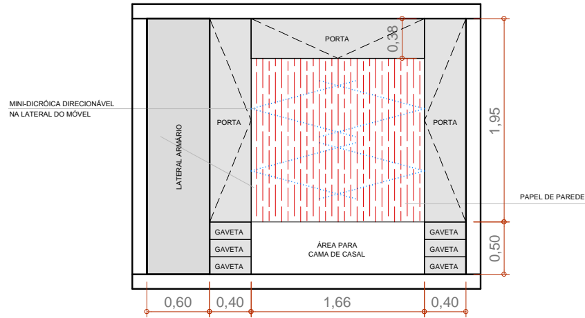
VISTA 01 ESCALA 1:50
