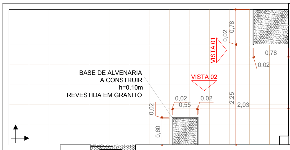
PLANTA ÁREA EXTERNA ESCALA 1:50
