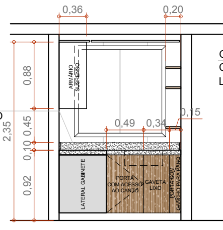
VISTA 02 ESCALA 1:50
