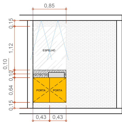
VISTA BANHEIRO ESCALA 1:50
