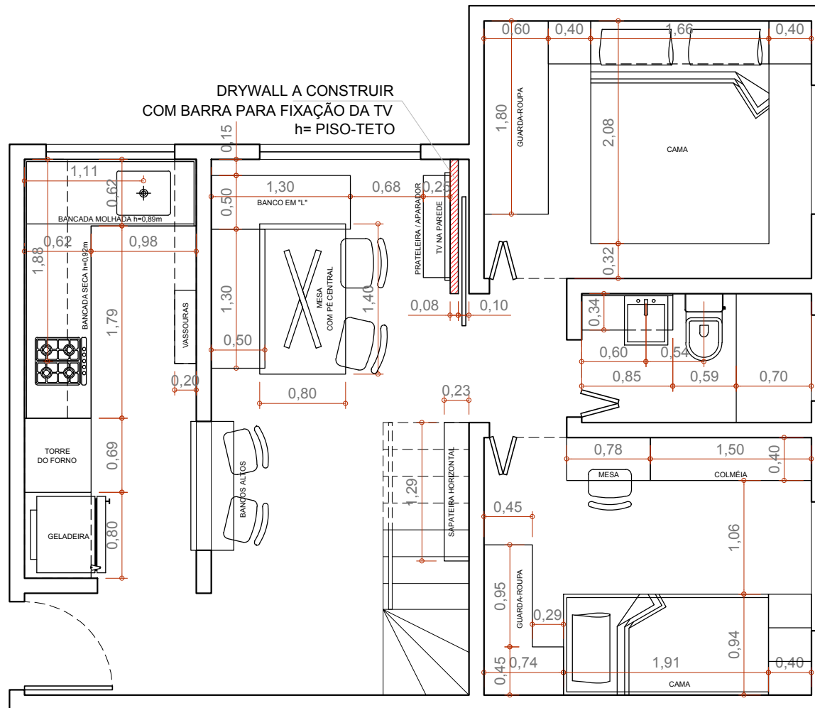
PLANTA PAV. INFERIOR ESCALA 1:50
