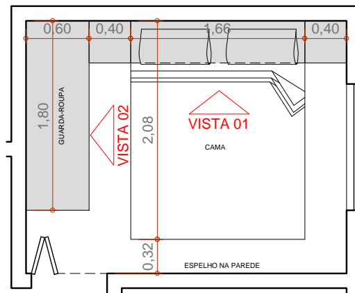
PLANTA ESCALA 1:50
