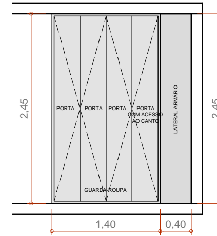
VISTA 02 ESCALA 1:50
