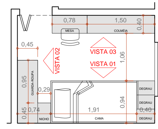
PLANTA ESCALA 1:50
