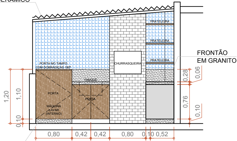
VISTA 01 ESCALA 1:50
