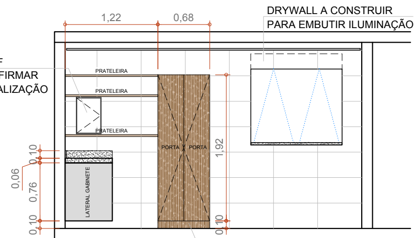
VISTA 03 ESCALA 1:50
