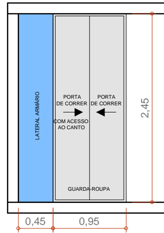
VISTA 02 ESCALA 1:50
