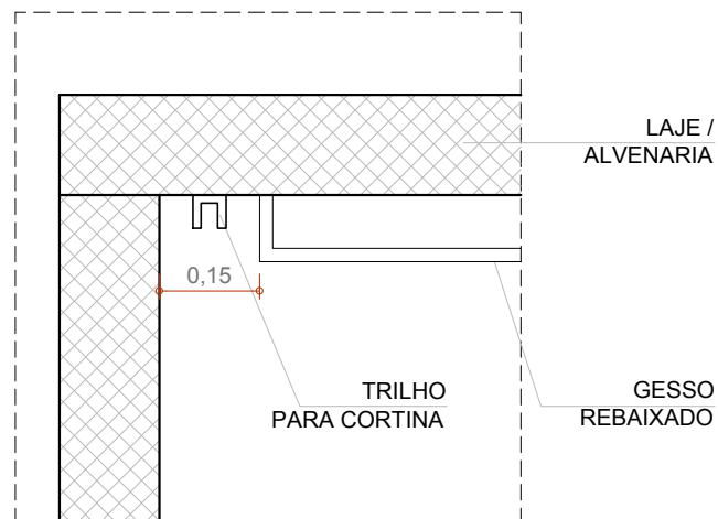
DETALHE 02 TRILHO DA CORTINA ESCALA 1:25
