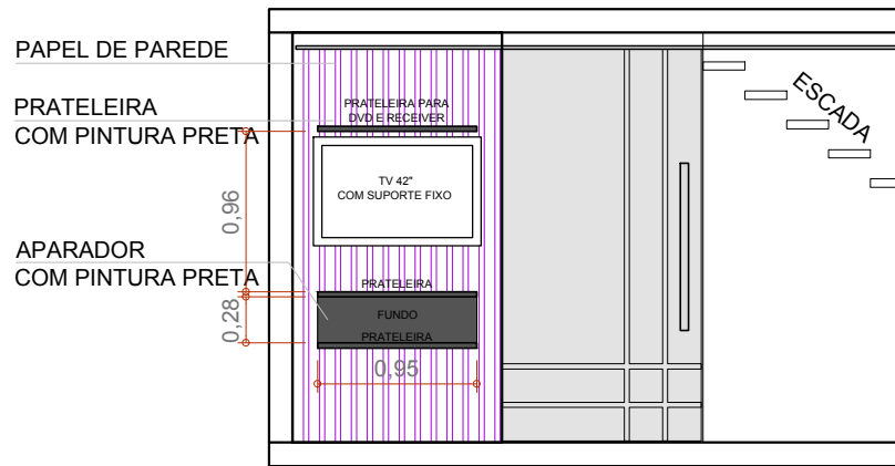
VISTA 01 ESCALA 1:50
