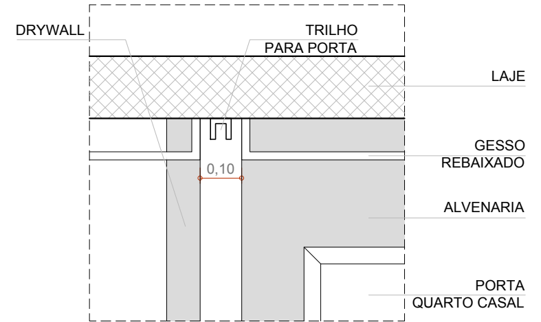
DETALHE 01 TRILHO DA PORTA DE CORRER ESCALA 1:25
