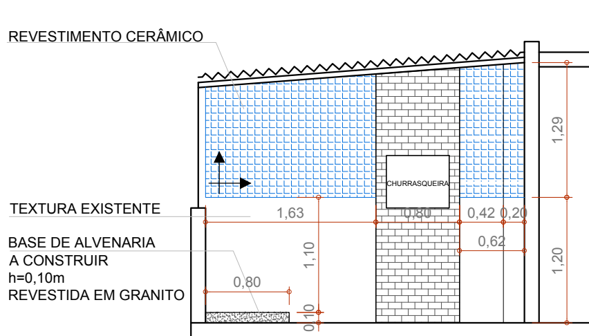
VISTA 01 ESCALA 1:50
