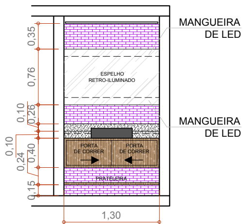
VISTA LAVABO ESCALA 1:50
