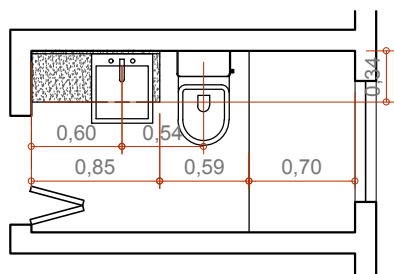
PLANTA BANHEIRO ESCALA 1:50
